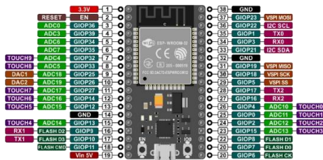
Gambar 4. ESP32
