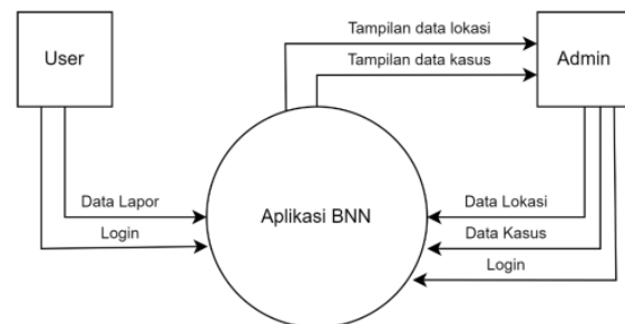
Gambar 1. Diagram Konteks
