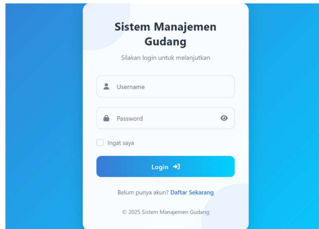
Gambar 4. Halaman login
