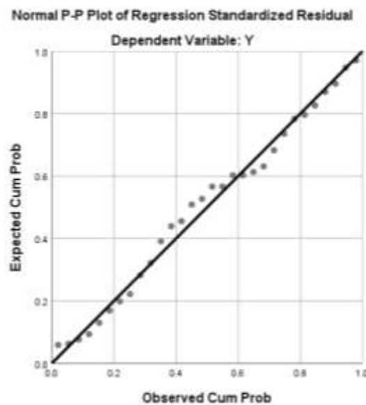
Grafik 1. Hasil uji normalitas
