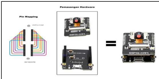
Gambar 15: Skema Rangkaian Esp32-Cam
