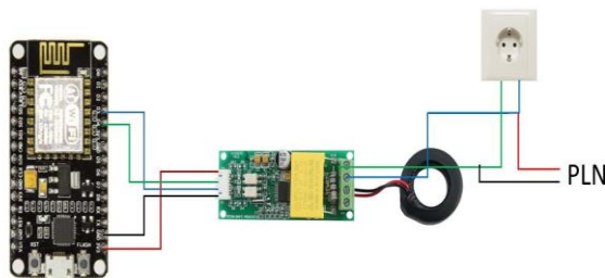
Gambar 16: Skema Rangkaian sensor PZEM004T
