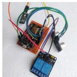
Gambar 9. Modul NodeMCU ESP8266 Dengan Relay
