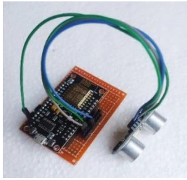
Gambar 7. NodeMCU ESP8266 Dengan Sensor Ultrasonik
